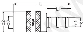
Муфта под шланг с безхомутвым соединением / Hose Clamp Socket
