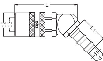
Муфта 45° под шланг с безхомутвым соединением / 45° Hose Clamp Socket
