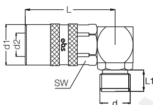
Муфта 90° с наружной резьбой / 90° Male Socket
