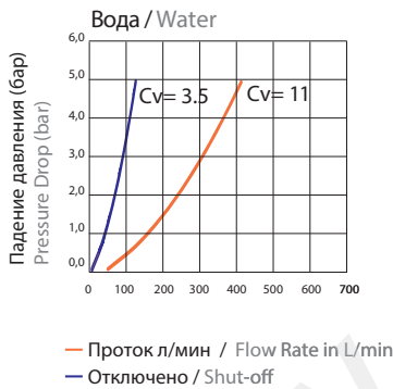
График зависимости протока от падения давления Flow Rate vs Pressure Drop Graph
