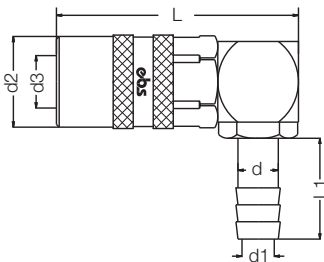
Муфта под шланг с безмоутовым соединением / Hose Clamp Socket
