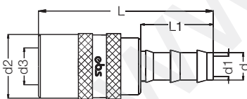
Муфта под шланг с безмоутовым соединением / Hose Clamp Socket
