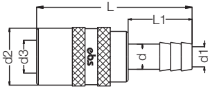
Муфта прямая под шланг / Hose Tail Socket
