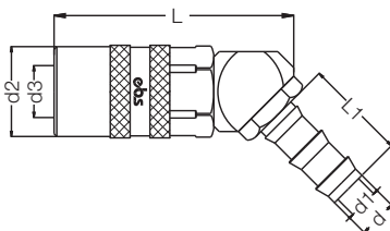
Муфта 45° под шланг с безмоутовым соединением / 45° Hose Clamp Socket
