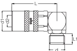
Муфта 90° с наружной резьбой / 45° Male Socket
