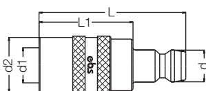
Адаптер муфты / Adapting Socket with Plug
