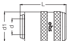
Адаптер муфты / Adapter Socket
