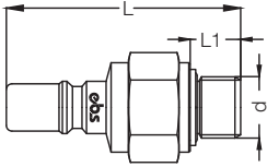
Ниппель с внешней резьбой / Male Plugs
