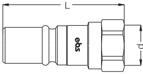
Ниппель с внутренней резьбой / Female Plugs
