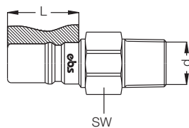
Ниппель с наружной резьбой / Female Plugs
