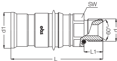
Муфта с наружной резьбой / Male Thread Socket
