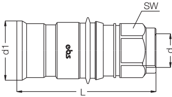
Муфта с внутренней резьбой / Female Thread Socket
