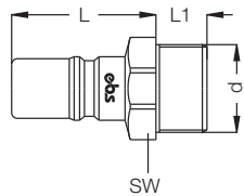
Ниппель с внешней резьбой / Male Plugs
