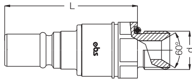
Ниппель с внешней резьбой / Male Plugs
