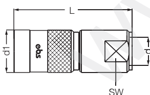
Муфта прямая с наружной резьбой / Male Thread Socket
