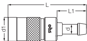
Муфта под шланг с безмоутовым соединением / Hose Clamp Socket
