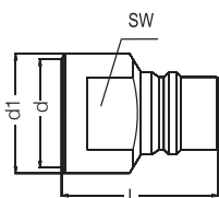
Ниппель с внутренней резьбой
