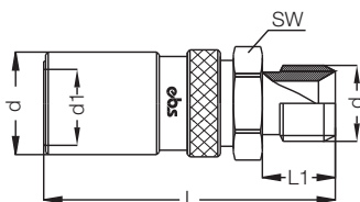
Муфта прямая с внешней резьбой / Male Socket
