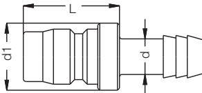
Ниппель с внешней резьбой / Male Plug
