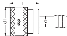
Ниппель под шланг / Hose Plugs
