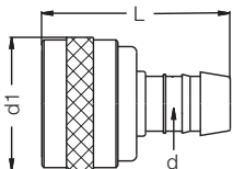
Муфта под шланг / Hose Tail Socket
