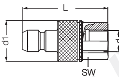
Ниппель с внешней резьбой / Male Plugs
