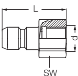
Ниппель с внутренней резьбой / Female Plugs
