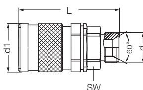
Муфта с внешней резьбой / Male Thread Socket
