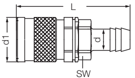
Муфта под шланг / Hose Tail Socket
