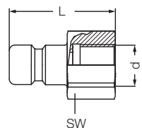
Ниппель с внутренней резьбой / Female Plugs
