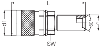
Муфта с внешней резьбой / Male Thread Socket
