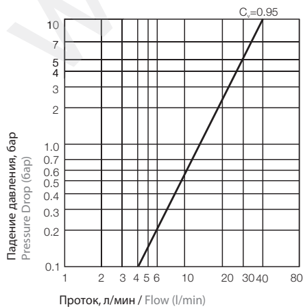
График зависимости протoka от падения давления / Flow Rate vs Pressure Drop Graph
