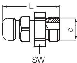
Ниппель с внешней резьбой / Male Plug
