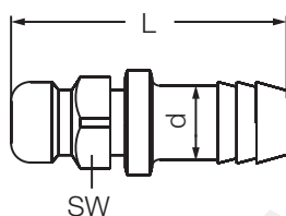
Ниппель под шланг / Hose Plug
