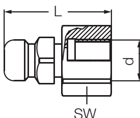
Ниппель с внутренней резьбой / Female Plug
