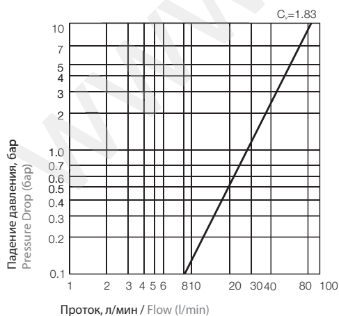
График зависимости протoka от падения давления / Flow Rate vs Pressure Drop Graph
