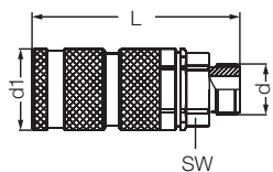
Муфта с внутренней резьбой / Female Thread Socket
