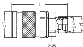
Муфта с внутренней резьбой / Female Thread Socket
