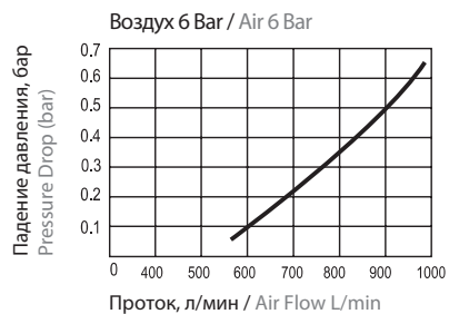
График зависимости потока от падения давления Flow Rate vs Pressure Drop Graph
