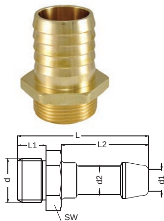
Ниппель с внешней резьбой Male Threaded Hose Tail
