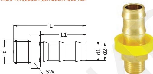
Ниппель с внешней резьбой под шланг с бесьомутовым соединением Push Lock Male Threaded Push Lock Hose Tail
