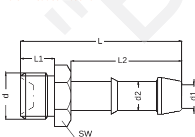
Ниппель с внешней резьбой Male Threaded Hose Tail
