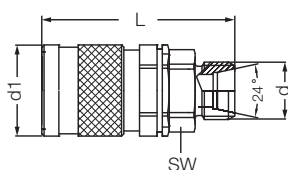
Муфта с внешней резьбой / Male Thread Socket
