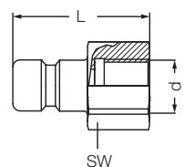
Ниппель с внутренней резьбой / Female Plugs
