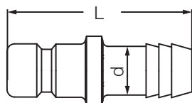
Ниппель под шланг / Hose Plugs
