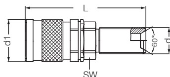
Муфта с внешней резьбой / Male Thread Socket
