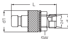
Ниппель с внешней резьбой / Male Plugs
