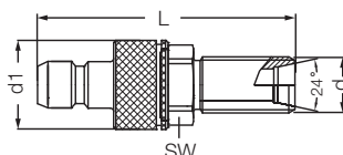
Ниппель с внутренней резьбой / Female Plugs
