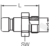
Ниппель с внутренней резьбой / Female Plugs
