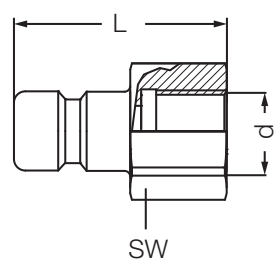
Ниппель с внутренней резьбой / Female Plugs
