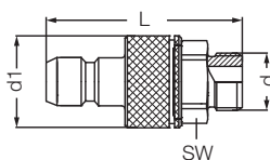
Ниппель с внешней резьбой / Male Plugs
