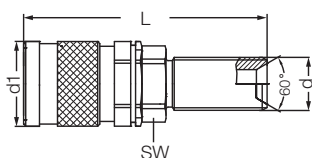
Муфта с внешней резьбой / Male Thread Socket
