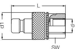
Ниппель под шланг / Hose Plugs
