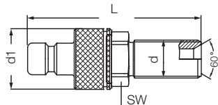
Ниппель с внешней резьбой / Male Plugs
