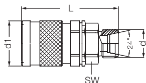
Муфта с внешней резьбой / Male Thread Socket
