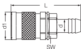
Муфта под шланг / Hose Tail Socket
