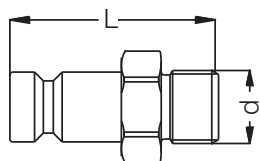
Ниппель с внешней резьбой / Male Plugs
