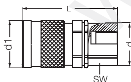
Муфта под шланг / Hose Tail Socket
