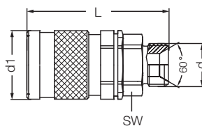
ЕМуфта с внешней резьбой / Male Thread Socket
