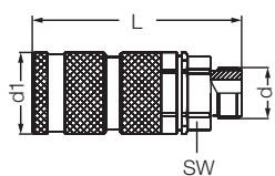
Муфта с внутренней резьбой / Female Thread Socket
