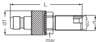
Ниппель с внешней резьбой / Male Plugs
