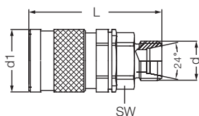
Муфта с внутренней резьбой / Female Thread Socket
