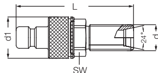
Ниппель с внутренней резьбой / Female Plugs
