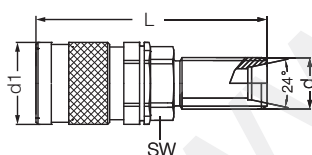
Муфта с внутренней резьбой / Female Thread Socket
