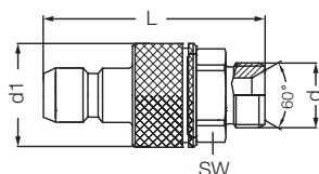
Ниппель с внешней резьбой / Male Plugs
