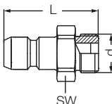
Ниппель с внутренней резьбой / Female Plugs
