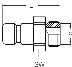
Ниппель с внешней резьбой / Male Plugs
