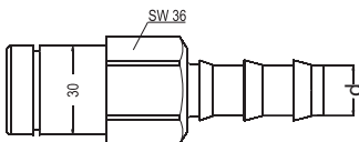
Муфта под шланг с безхомутным соединением Push-lock
