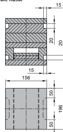
Зажимные пазы
